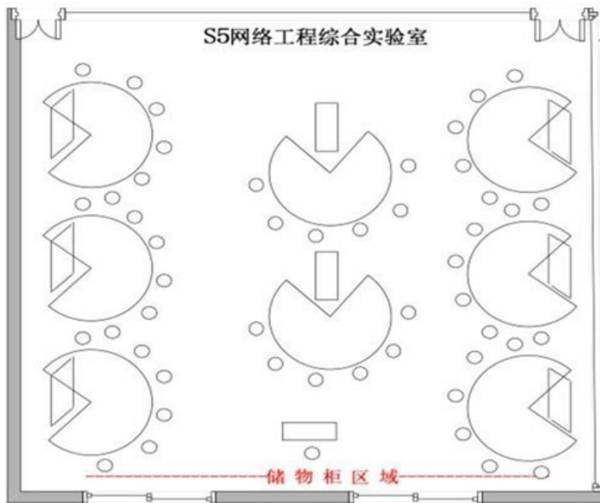
Remark: Construction area : 13.4×12.3=164.82 m 2
